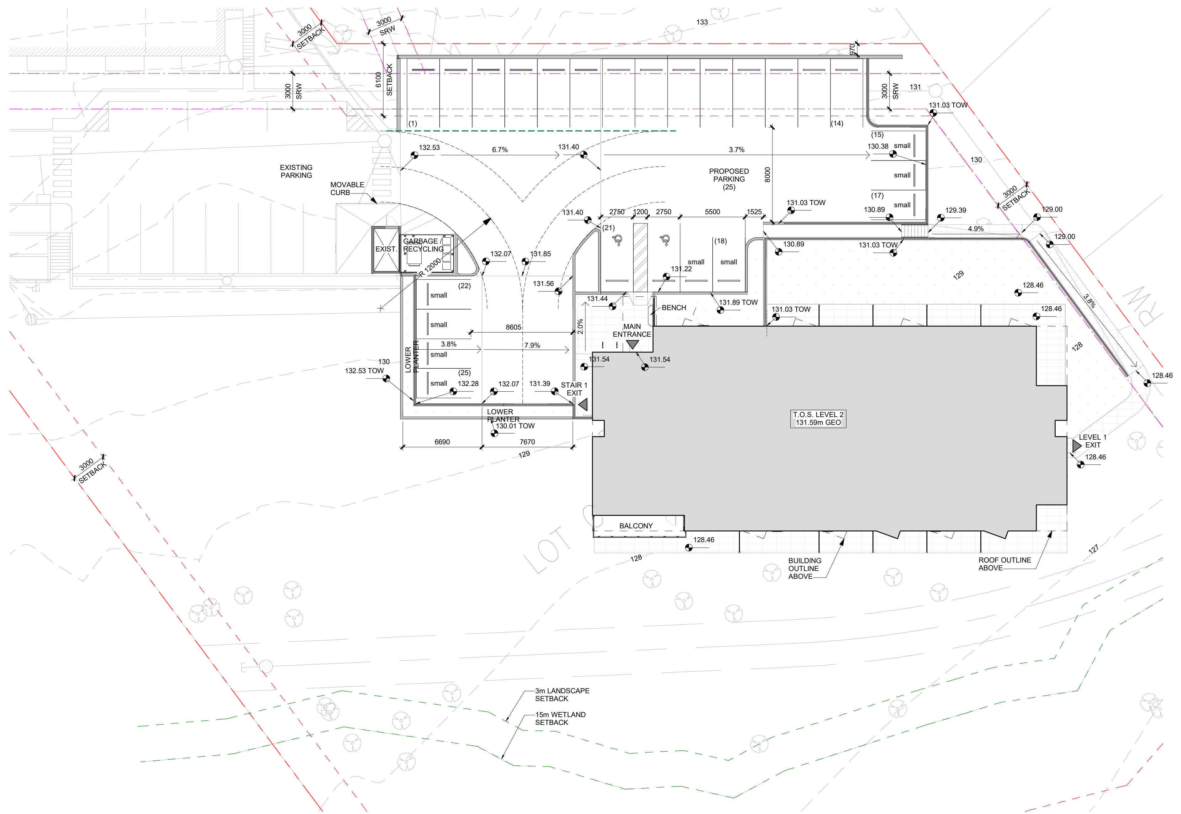
1 D05 SITE PLAN D05 1:200
