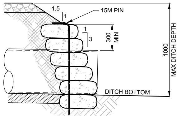
SECTION 1:25
